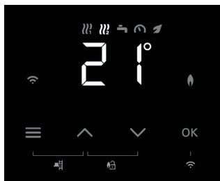
7-segmenses LCD kijelző érintő gombokkal
